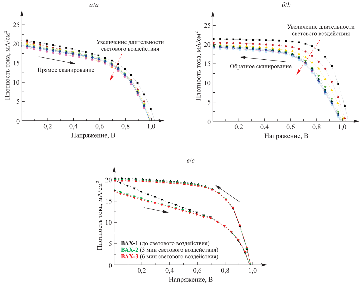
Рис. 1. Световые ВАХ ПСЭ, измеренные при прямом (а) и обратном (б) направлениях сканирования, а также после темнового восстановления и последующего светового воздействия (в)
