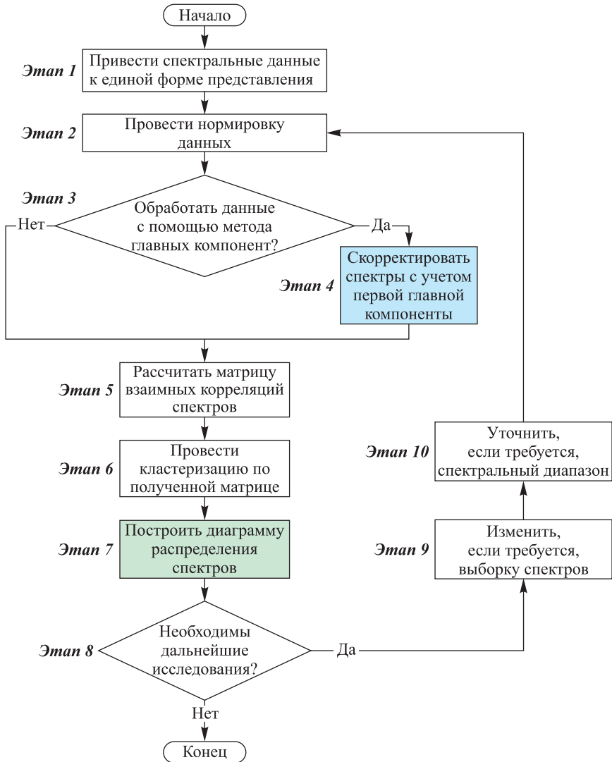
Рис. 2. Структурная схема разработанного алгоритма классификации
