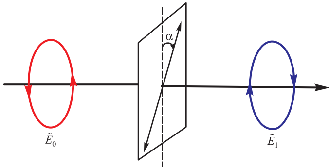
Рис. 3. Нормальное прохождение циркулярно поляризованного света \tilde{E}_0 через полуволновую фазовую пластину, повернутую под некоторым углом \alpha
