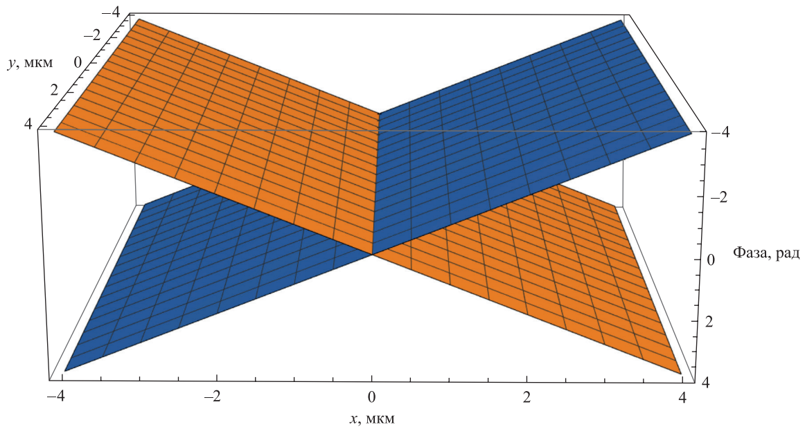
Рис. 6. Профиль поверхности геометрической фазы для поляризационной дифракционной ЖК-решетки
