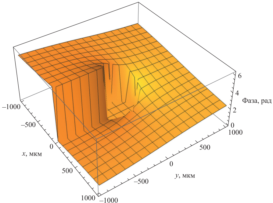
Рис. 17. Фазовая поверхность q -пластины с фазовым ядром ( q = 0,5 , \sigma = 1 , r_0 = 0,25 мм)
