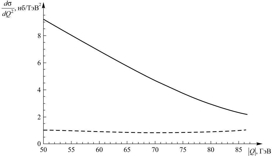
Рис. 3. Зависимость ковариантного дифференциального сечения рассеяния от передачи импульса для различных совокупностей вкладов.
