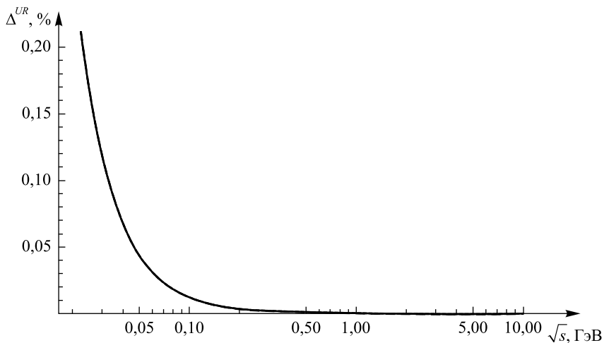
Рис. 8. Отличие сечения процесса, вычисленного в ультррелятивистском приближении, от его точного выражения в борновском приближении. Сплошной линии соответствует угол 0^\circ , штриховой – угол 5^\circ , точечной – угол 10^\circ
