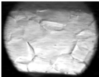
Рис. 3. Изменения полированной поверхности сплава \text{PdH}_{0.12} , инициированные повышением давления при T = 250^\circ\text{C} = \text{const.} . Время от начала приповерхностных изменений: a – 0 с; б – 1 с; в – 7 с
