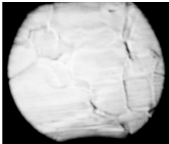
Рис. 4. Изменения полированной поверхности сплава \text{PdH}_{0.17} , инициированные повышением давления при T = 270^\circ\text{C} = \text{const} . Время от начала приповерхностных изменений: a – 0 с; б – 1 с; в – 2 с; г – 5 с
