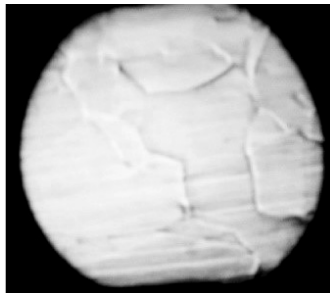
Рис. 4. Изменения полированной поверхности сплава \text{PdH}_{0.17} , инициированные повышением давления при T = 270^\circ\text{C} = \text{const} . Время от начала приповерхностных изменений: a – 0 с; б – 1 с; в – 2 с; г – 5 с
