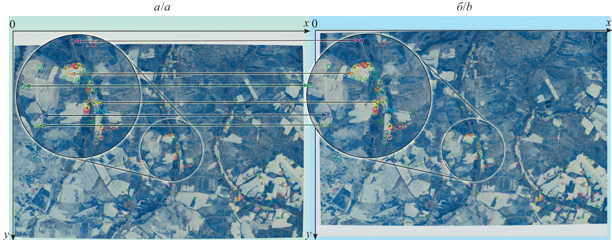
Рис. 1. Сопоставление двух изображений с выделением особых точек (детектором ORB): а – нетрансформированное изображение; б – трансформированное изображение
