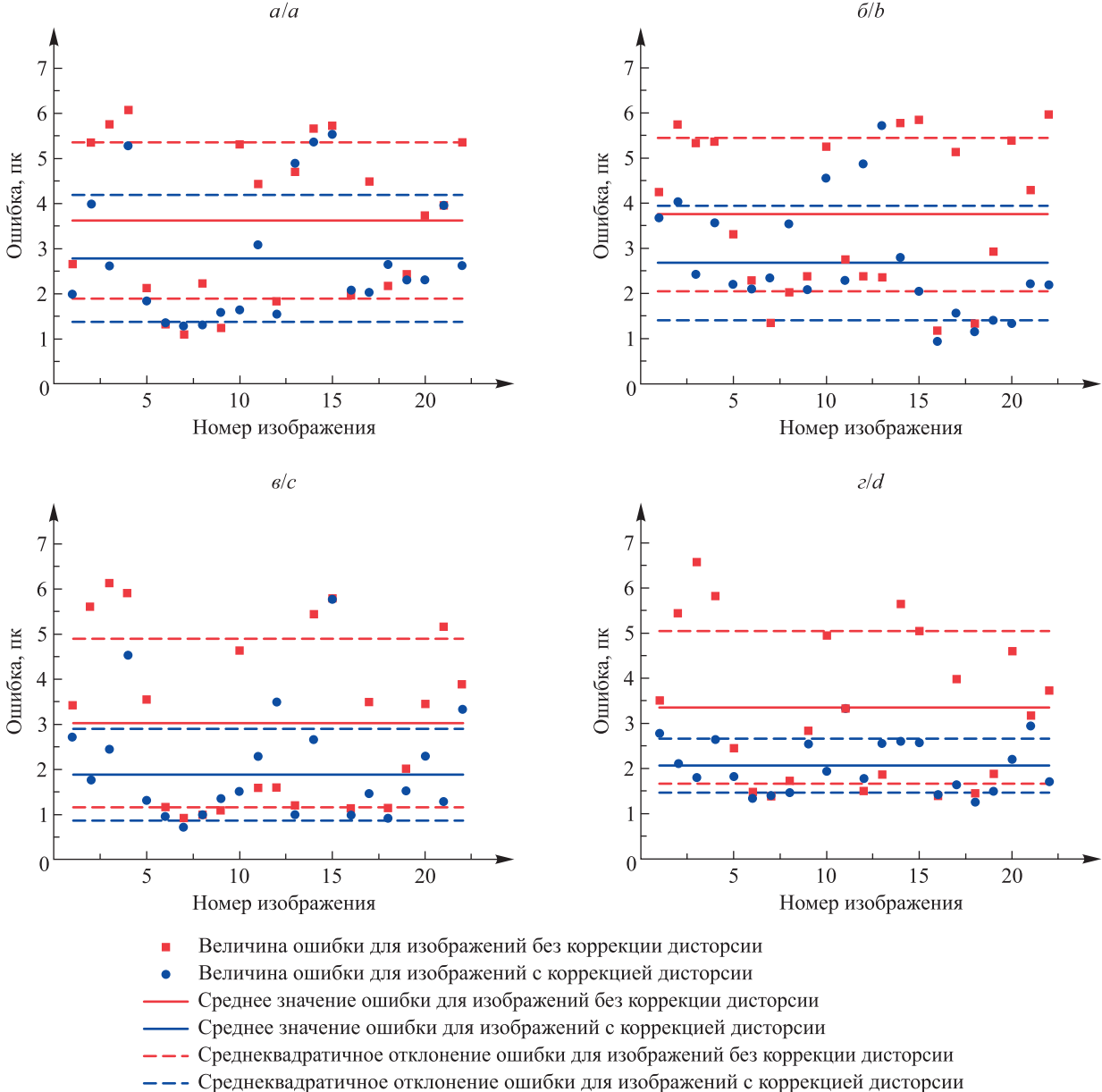
Рис. 2. Ошибки комбинирования для ряда изображений с коррекцией дисторсии и без нее при использовании различных детекторов и вычислителей дескрипторов: a – BRISK; b – Star + FREAK; c – ORB; d – ORB + FREAK
