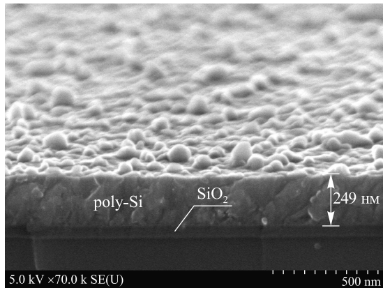
Рис. 1. РЭМ-изображение поверхности поликремния в структуре Al/poly-Si/SiO 2 /Si с удаленной пленкой алюминия сразу после ее напыления:
