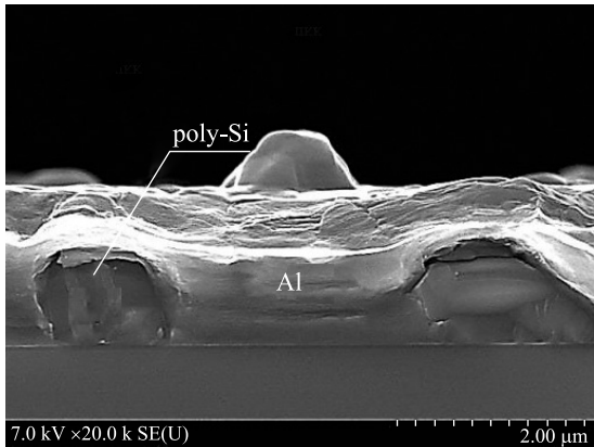
Рис. 2. РЭМ-изображение поперечного сечения структуры Al/poly-Si/SiO 2 /Si после длительной термообработки (450 °С, 20 мин)
