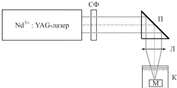
Рис. 1. Схема экспериментальной установки: СФ – светофильтр марки СЗС-23; П – поворотная призма; Л – фокусирующая линза ( f = 614 мм); К – кварцевая кювета с дистиллированной водой; М – мишень (металл)
