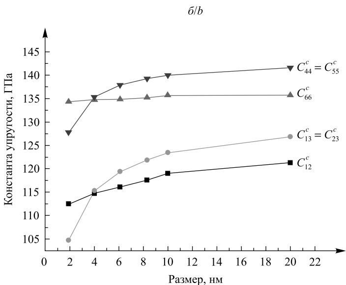
Рис. 3. Зависимость компонент тензора упругих констант столбчатых TiN-нанокристаллов от размера: a - C_{11}^c, C_{33}^c ; b - C_{12}^c, C_{13}^c, C_{44}^c, C_{66}^c
