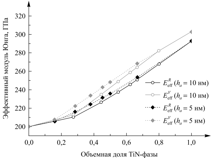
Рис. 5. Зависимость эффективного модуля Юнга слоистого TiN/Si 3 N 4 -нанокompозита от соотношения толщин слоев
