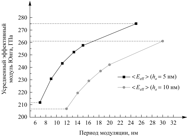
Рис. 6. Зависимость эффективного модуля Юнга слоистого \text{TiN}/\text{Si}_3\text{N}_4 -нанокompозита от периода модуляции
