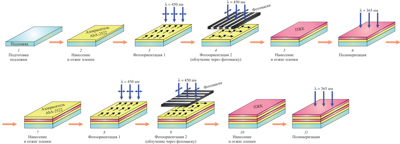
Рис. 2. Основные этапы (1–11) процесса изготовления многослойной дифракционной ЖК-структуры
