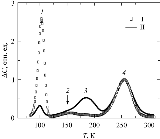
Рис. 3. Нормированные спектры DLTS ( \tau = 0,52 мс) для диодов Шоттки, облученных \gamma -квантами (I) и ионами H^+ (II). Цифрами 1–4 обозначены DLTS
