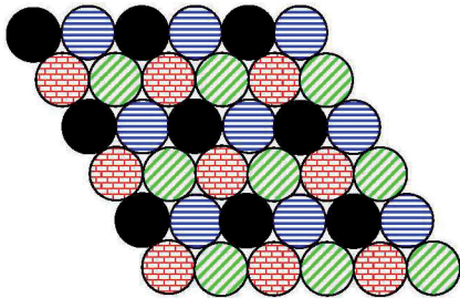
Рис. 3. Подрешеточная структура треугольной решетки с отталкиванием ближайших и притяжением третьих соседей.
