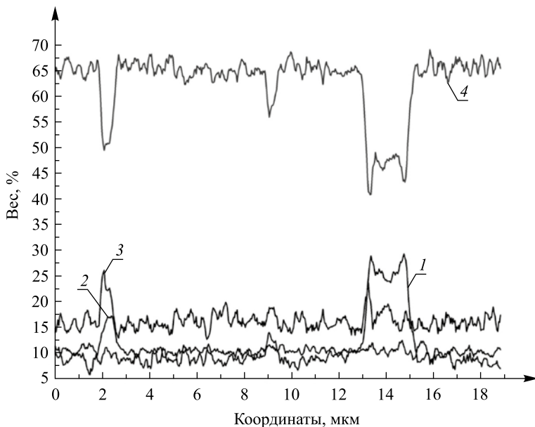
Рис. 2. РЭМ-изображение участка поверхности пленки Ag в \text{TiO}_2 на Si-подложке (а) и распределение элементного состава поверхности по линии на этом изображении (б): 1 – Ag; 2 – Ti; 3 – O; 4 – Si
