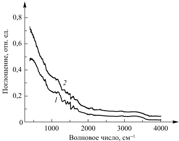
Рис. 1. Спектры НПВО пленок ФП9120 ( h = 1,0 мкм): 1 – исходных; 2 – имплантированных
