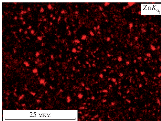
Рис. 2. Микроструктура (а) и карты распределений олова (б), цинка (в) и галлия (г) по поверхности приведенного участка микроструктуры
