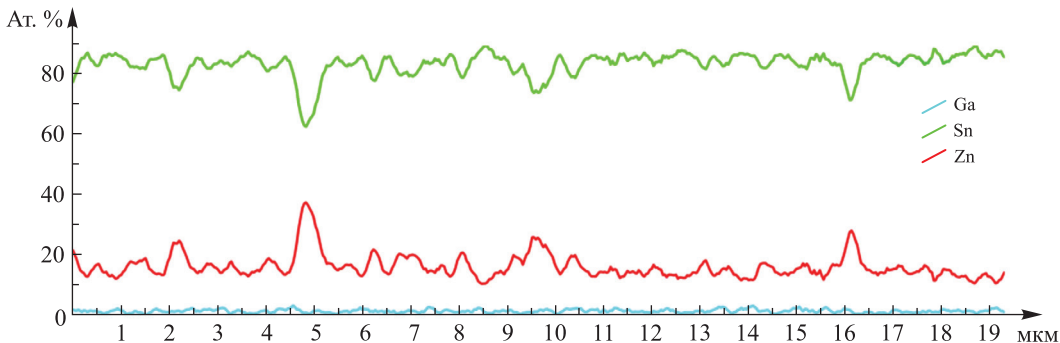
Рис. 3. Микроструктура (а) и распределение элементов вдоль линии сканирования L-L^I (б) поверхности А фольги сплава Sn – 10,8 ат. % Zn – 0,7 ат. % Ga
