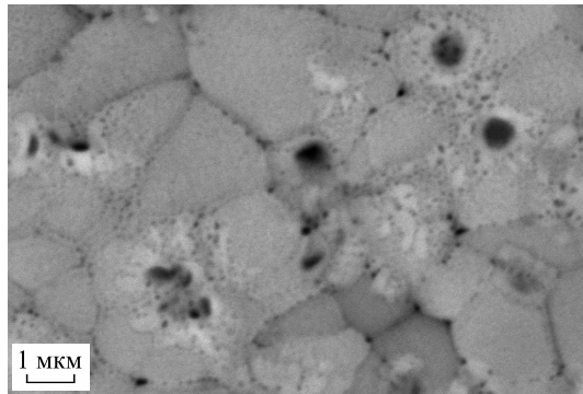
Рис. 4. Микроструктура участков поверхностей А (а) и В (б) фольги через 24 ч после ее изготовления
