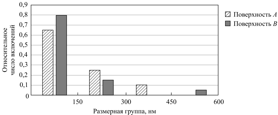
Рис. 5. Распределение включений цинка по размерным группам
