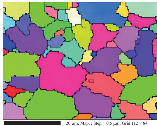
Рис. 8. Зеренная структура быстрозатвердевших фольг сплавов Sn – Zn – Ga околоэвтектического состава: a – поверхность A ; \delta – продольное сечение; \delta – поверхность B
