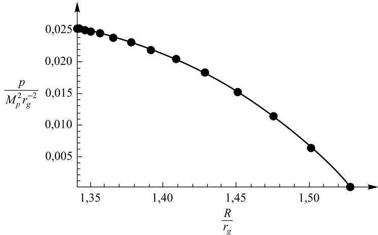
Рис. 6. Давление, полученное решением уравнения TOV (точки) и решением уравнений (4)–(7) (сплошная кривая). Численные значения параметров указаны в подписи к рис. 5, а, б
