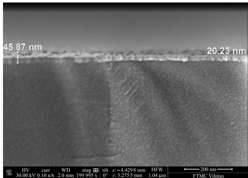
Рис. 3. СЭМ-изображения в поперечном направлении для образцов 1 (а) и 2 (б)
