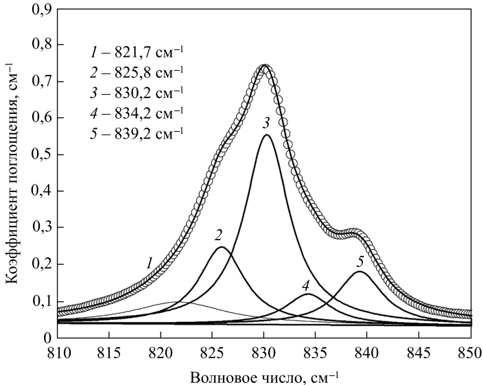
Рис. 3. Фрагмент спектра поглощения, измеренного при комнатной температуре, для образца Cz-Si ( [\text{O}_i] = 8,3 \cdot 10^{17} , [\text{C}_s] = 7 \cdot 10^{16} , [\text{P}] = 1 \cdot 10^{14} \text{ cm}^{-3} ), облученного нейтронами ( F = 7,5 \cdot 10^{16} \text{ cm}^{-2} ), после отжига при температуре 275 °C в течение 30 мин. Сплошные линии – подгонка с использованием функции Лоренца
