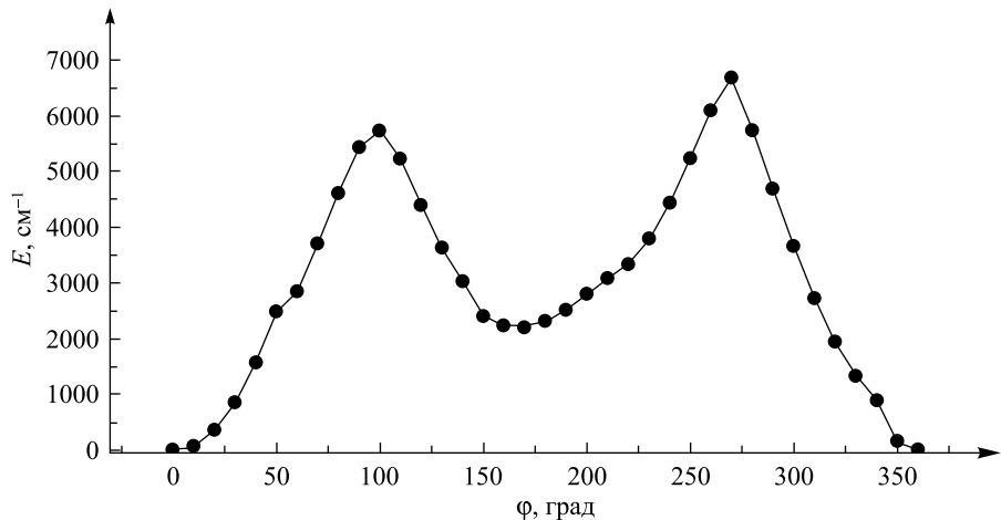
Рис. 2. Зависимость энергии основного состояния соединения Th-C11 от угла \phi
