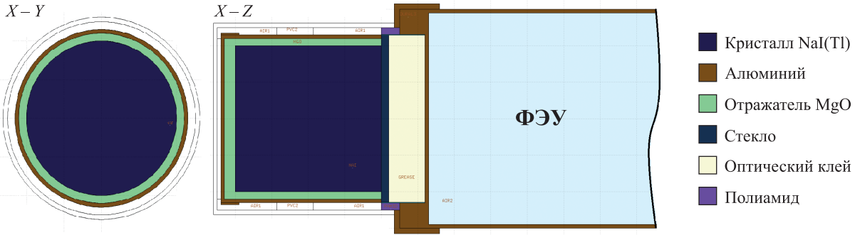
Рис. 1. Модель детектора БДКГ-05К с указанием основных конструкционных материалов
