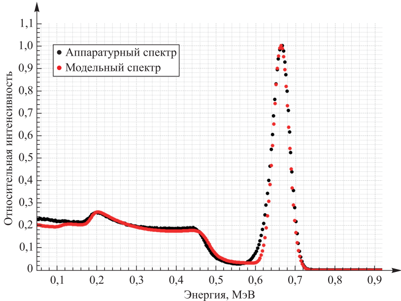
Рис. 2. Сравнение аппаратного и модельного спектров для радионуклида ^{137}\text{Cs} Fig. 2. Comparison of measured and modelled spectra of ^{137}\text{Cs} radionuclide
