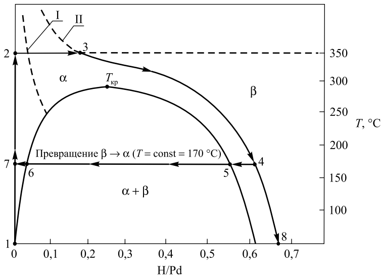
Рис. 1. Диаграмма состояния системы Pd – H и схемы водородных обработок:
