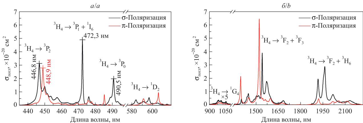
Рис. 4. Спектры сечения поглощения кристалла Pr : YAB в поляризованном свете в видимой (а) и инфракрасной (б) областях спектра
