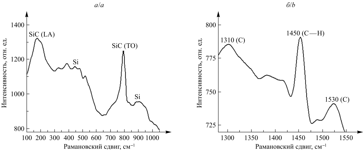
Рис. 3. Спектр КРС структуры SiC/Si, измеренный в области частот колебаний: a – связей Si—C; b – связей C—C
