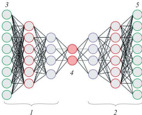
Рис. 3. Модель сверточного автоэнкодера:
