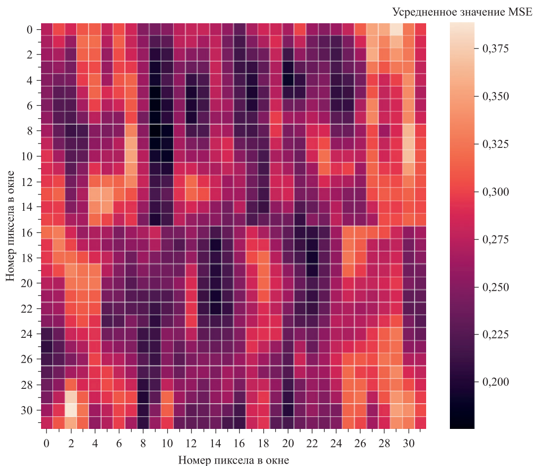
Рис. 7. Распределение средноквадратичной ошибки предсказания по областям изображения
