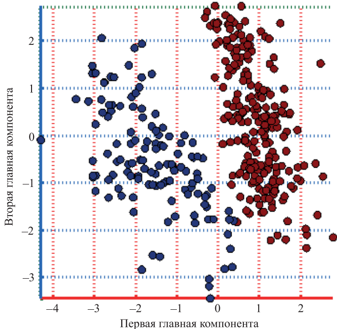
Рис. 5. Первичная классификация всей лабораторной спектральной выборки. Здесь и далее разные цвета соответствуют разным автоматически выделенным классам
