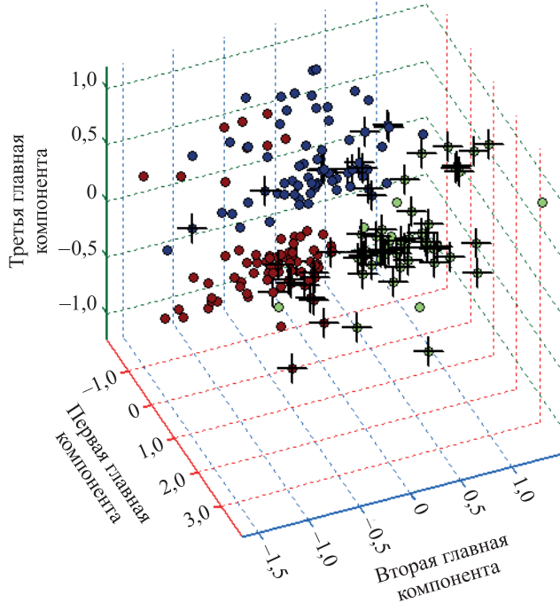
Рис. 8. Результат классификации PCA – pure – without 1 st – ward – seuclidian – 700–869.5 nm.
