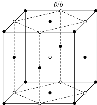
Рис. 1. Кубическая решетка с ячейкой F -типа (а) и построенная на ее основе ячейка I -типа (б)
