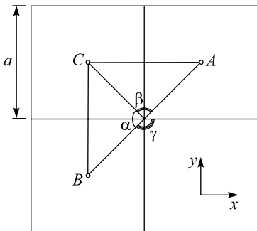
Рис. 2. Переход от ячейки I -типа к ячейке P -типа. \vec{AB}\vec{BC} – базис ячейки P -типа
