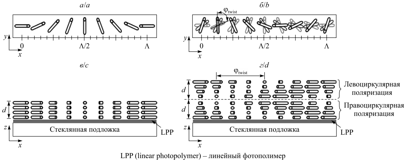
Рис. 4. Базовая геометрия поляризационной решетки (а – вид сверху; в – вид сбоку). Ахроматическая поляризационная решетка с двумя хиральными слоями ЖК с разным знаком закрутки (б – вид сверху; г – вид сбоку). Источник: [15]
