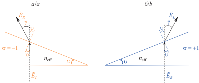
Рис. 8. Оптические схемы модели эквивалентной призмы для левоциркулярно поляризованного (а) и правоциркулярно поляризованного (б) света, нормально падающего на поляризационную дифракционную ЖК-решетку
