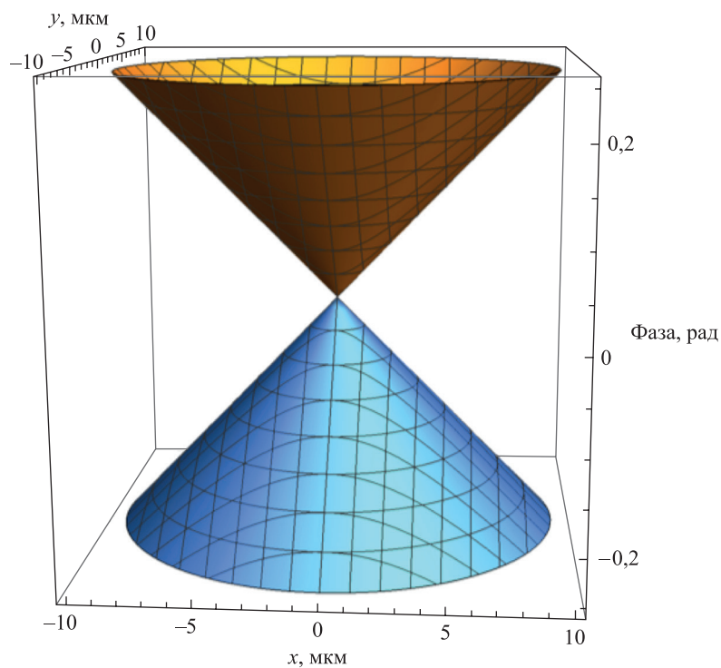
Рис. 11. Фазовая поверхность кольцевой решетки (\Lambda = 120 \text{ мкм}, \lambda = 1,55 \text{ мкм})
