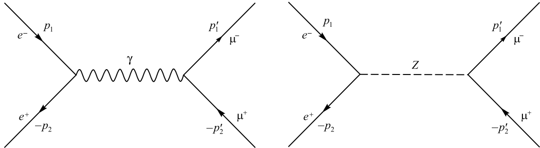
Рис. 1. Диаграммы процесса e^- e^+ \rightarrow \mu^- \mu^+ в борновском приближении Fig. 1. Diagrams of the e^- e^+ \rightarrow \mu^- \mu^+ process in the Born approximation
