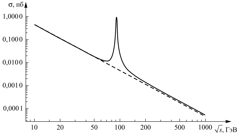
Рис. 5. Полное сечение процесса рассеяния для различных совокупностей вкладов.
