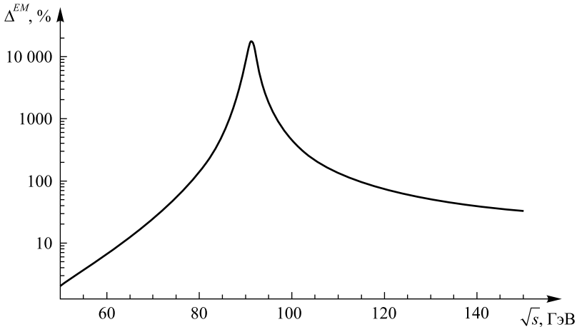
Рис. 6. Относительная разность полного и электромагнитного вкладов
