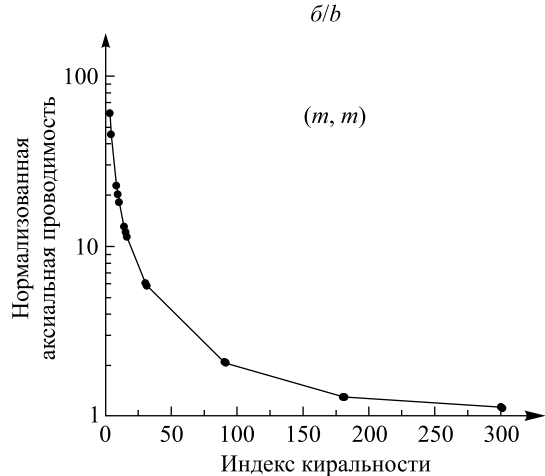
Рис. 1. Нормированная на проводимость графита аксиальная проводимость нанотрубок типа zigzag (a) и armchair (b).
