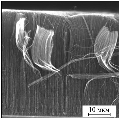
Рис. 2. Массив вертикально ориентированных многослойных УНТ. Изображения получены с помощью растрового микроскопа ( а ) и просвечивающего электронного микроскопа ( б ).
